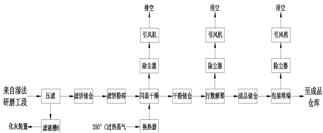
图 5-5 碳酸钙生产：干燥、解聚、包装工序流程图
