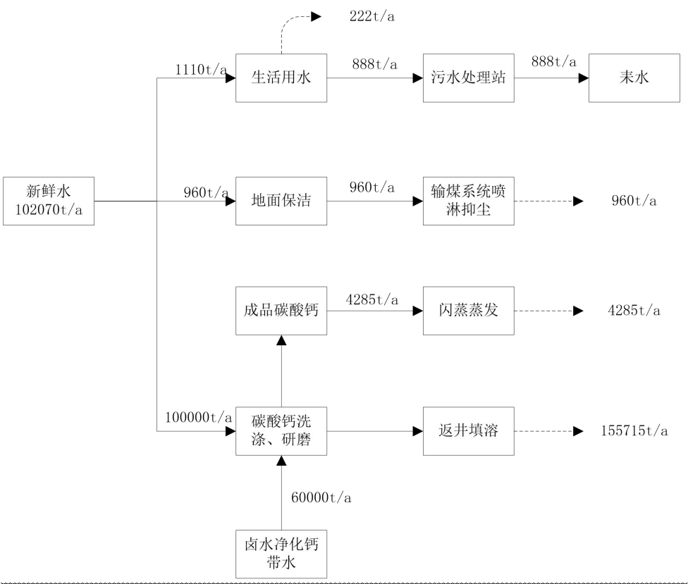
图5-5 项目水平衡图
