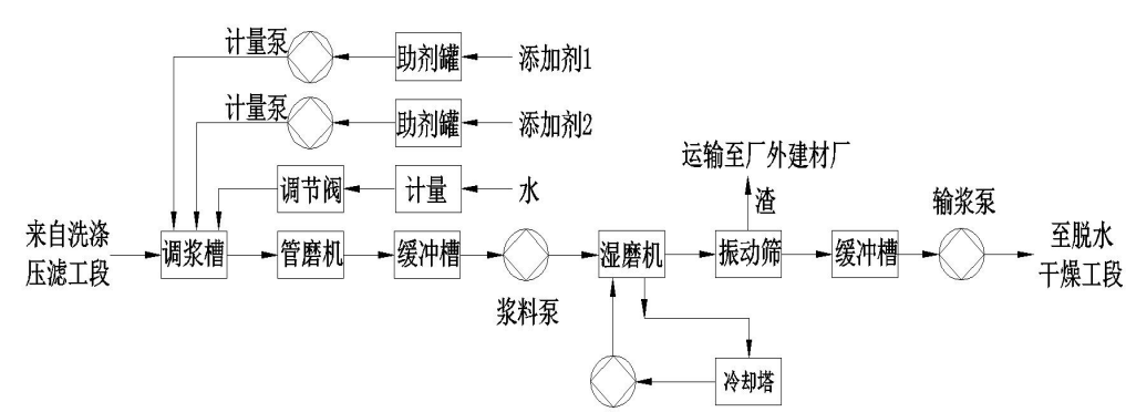
图 5-4 碳酸钙生产：研磨工序流程图
