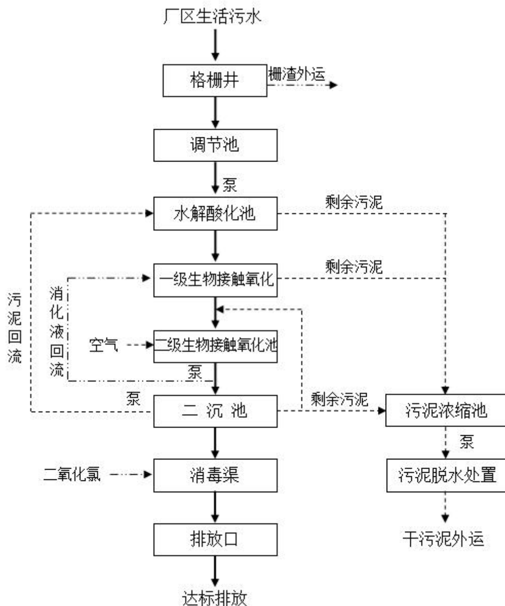
图 7-1 厂区污水处理站工艺流程
