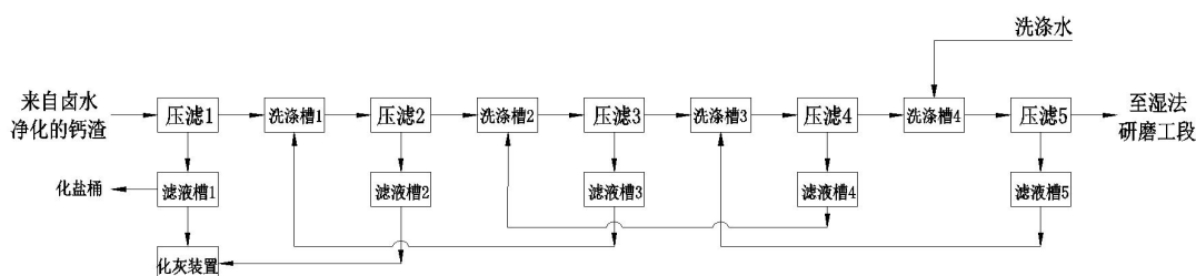
图 5-3 碳酸钙生产：洗涤工序流程图
