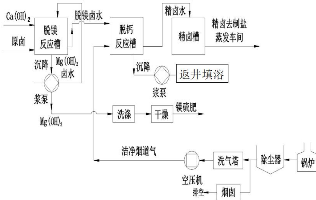
图 1-1 现有卤水净化工段工艺流程图
